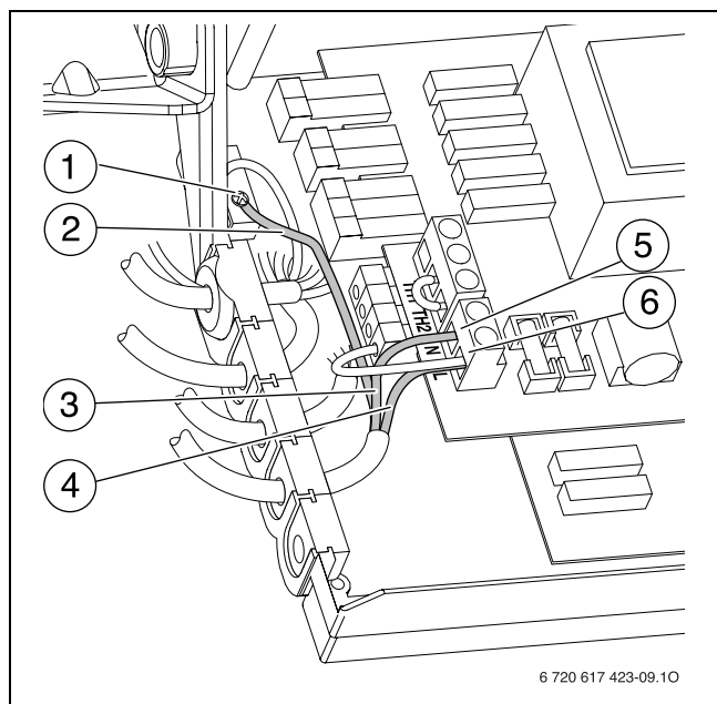
Fig. 26 Collegamento cavo 230 V AC
