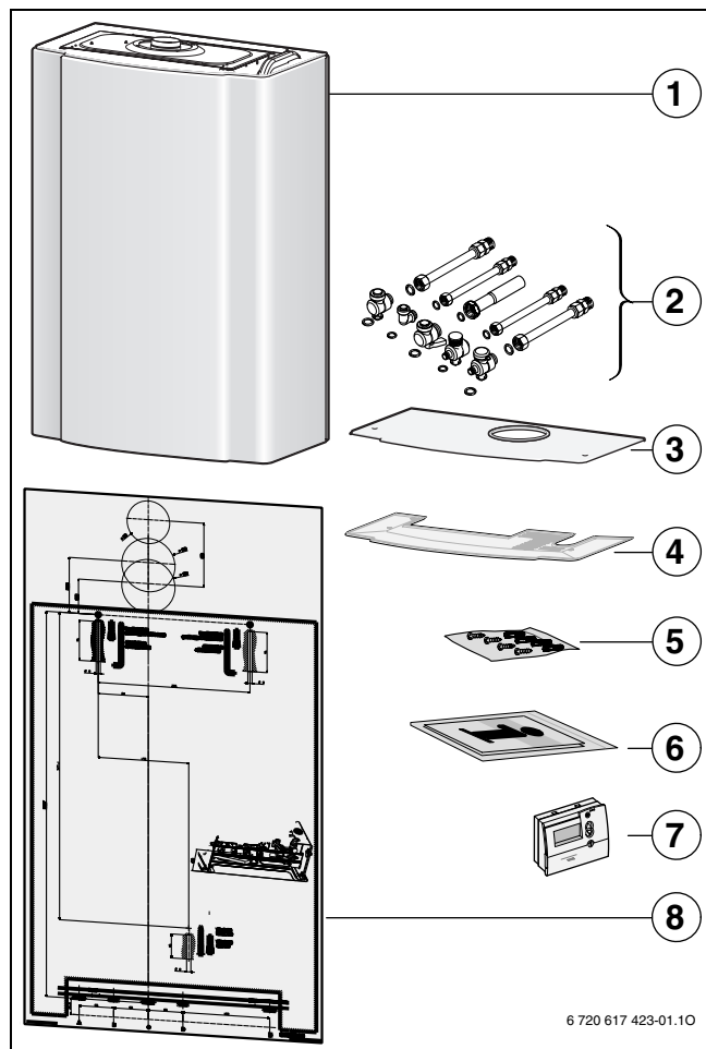
Fig. 1 ZWA 24/28-2/3 AB
