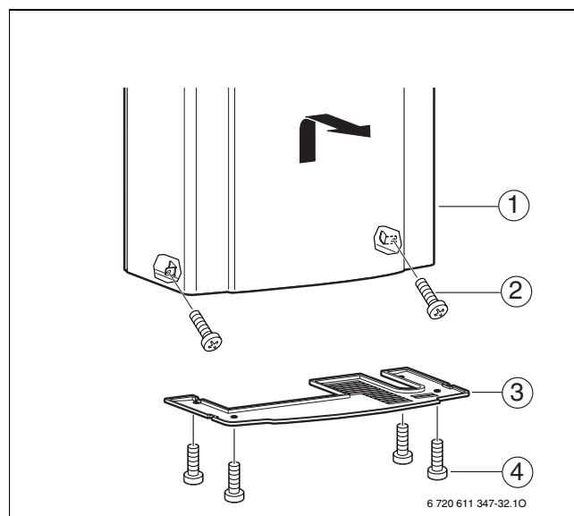
Fig. 44 Rimuovere la copertura inferiore e il rivestimento
