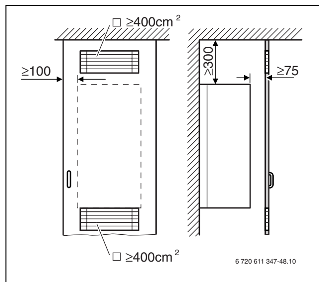
Fig. 9 Aperture di aerazione per il montaggio in un armadio
