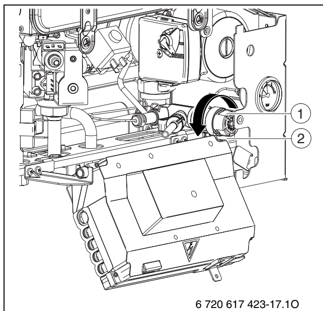
Fig. 51 Valvola di sicurezza riscaldamento
