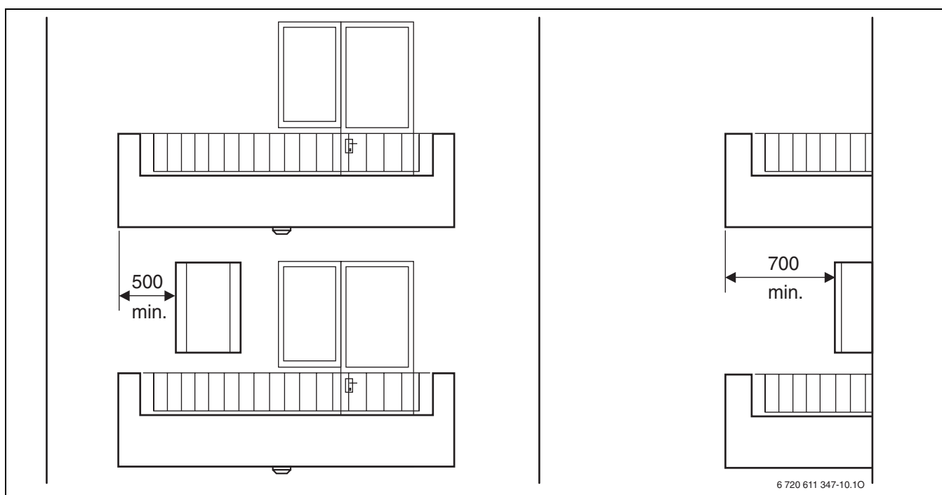
Fig. 4 Protezione minima necessaria
