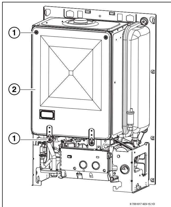
Fig. 45 Aprire la camera stagna
