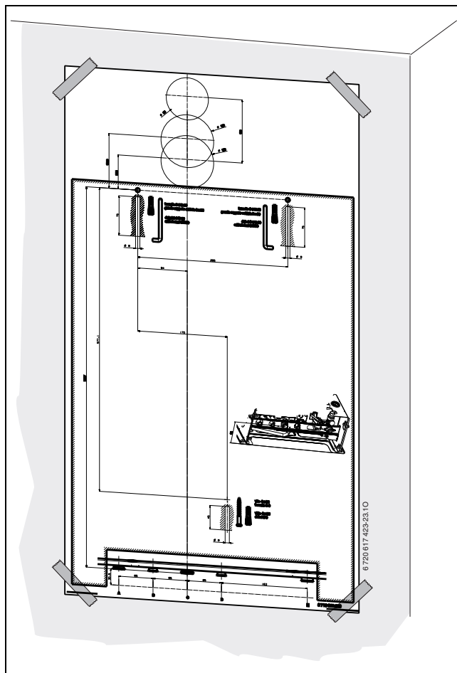
Fig. 10 Fissaggio a muro della dima di montaggio.
