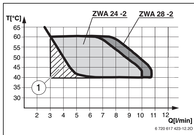
Fig. 34 Diagramma per una temperatura in entrata dell'acqua fredda di +10 °C
