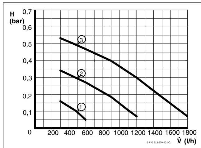
Fig. 33 Diagramma delle curve caratteristiche/velocità del circolatore
