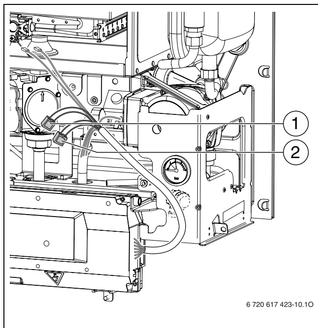
Fig. 27 Collegamenti nell'apparecchio
