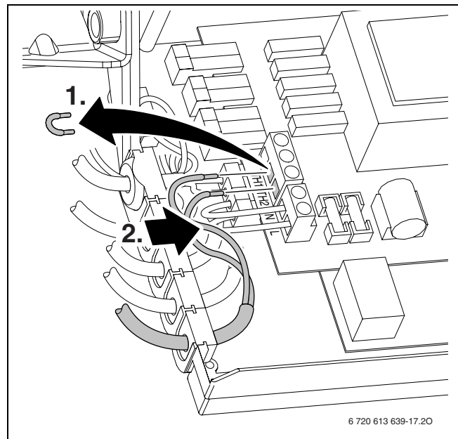
Fig. 25 Collegamento (230 V CA, rimuovere il ponticello tra TH1 e TH2)
