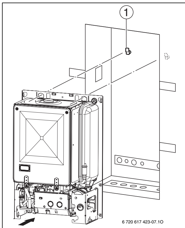
Fig. 13 Fissaggio a muro nel guscio per incasso
