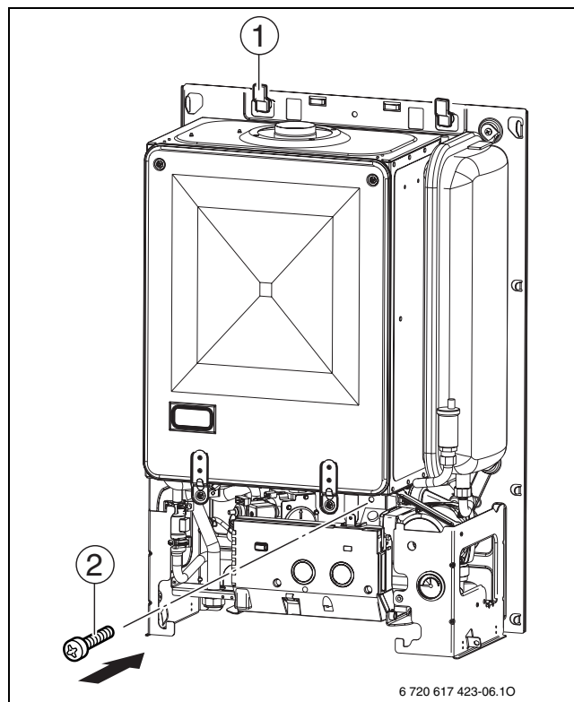
Fig. 12 Fissaggio a muro
