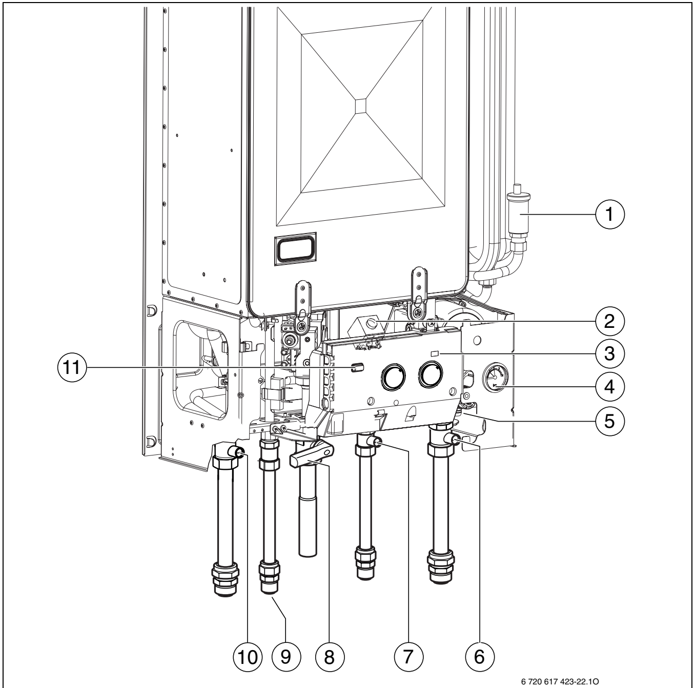
Fig. 28 Caldaia raffigurata, ZWA ...-2/3 AI
