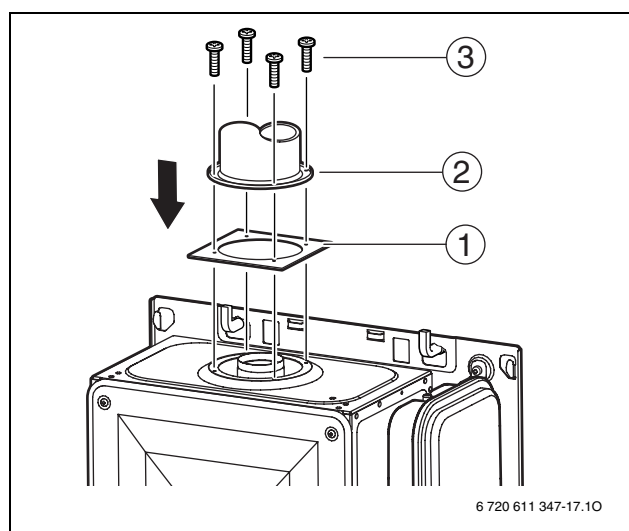
Fig. 18 Fissaggio dell'accessorio per gas combusti (esempio Ø 80 mm)
